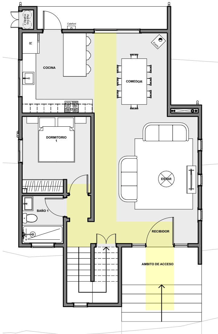
PLANTA DE ARQUITECTURA 1° PISO 1:100
