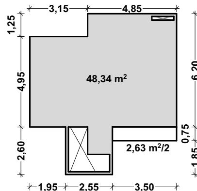
ESQUEMA DE SUP. 2° PISO 1:200
