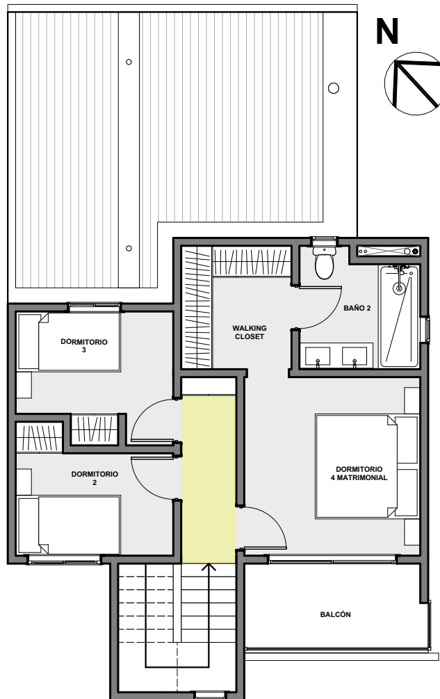
PLANTA DE ARQUITECTURA 2° PISO 1:100
