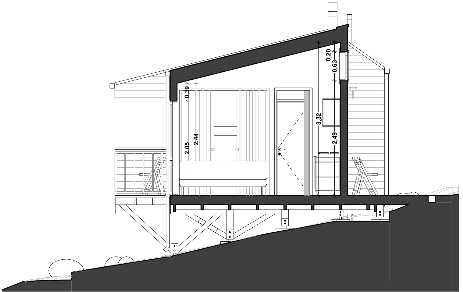
Corte B - B 1:50
