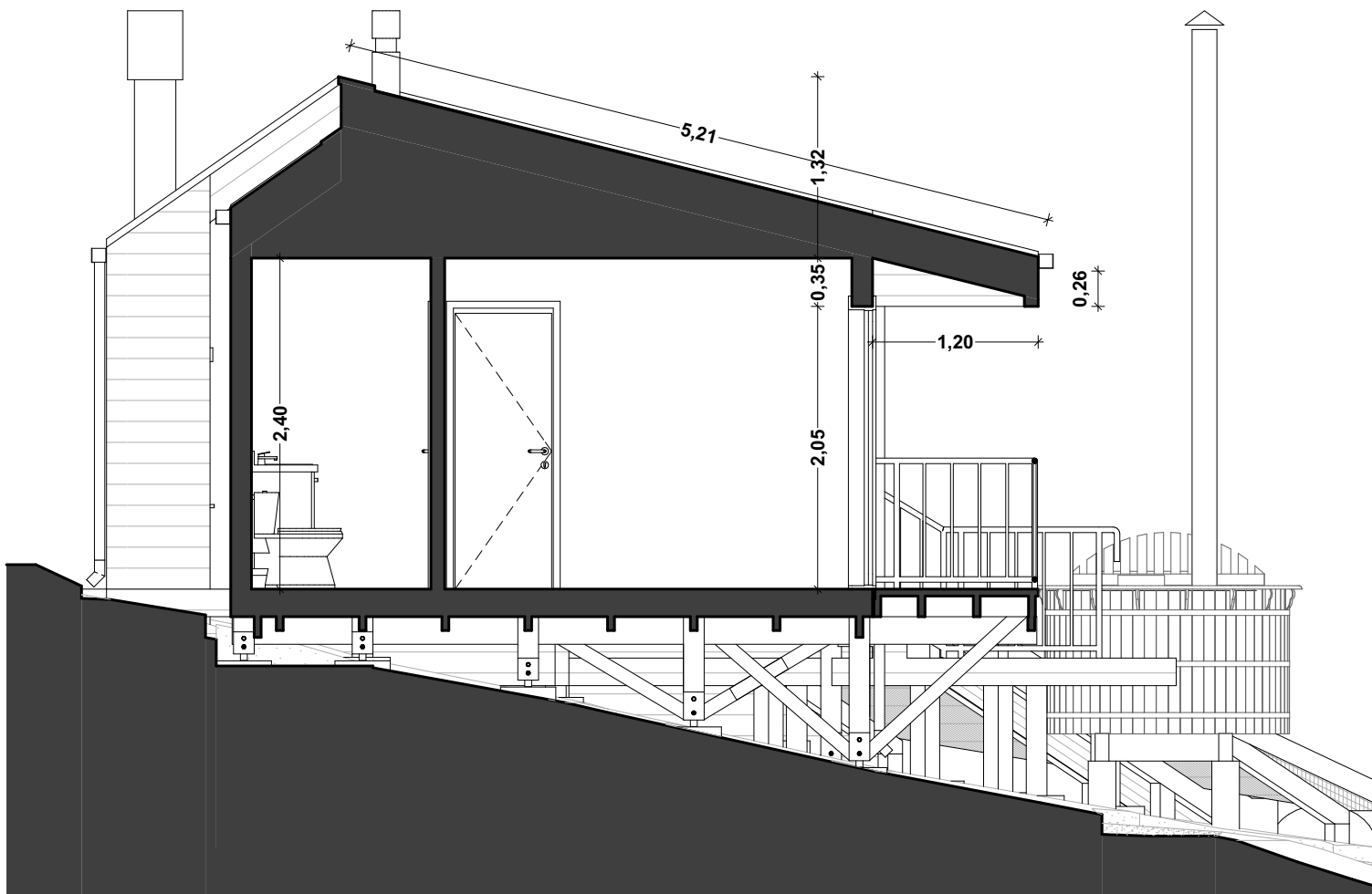
Corte D - D 1:50
