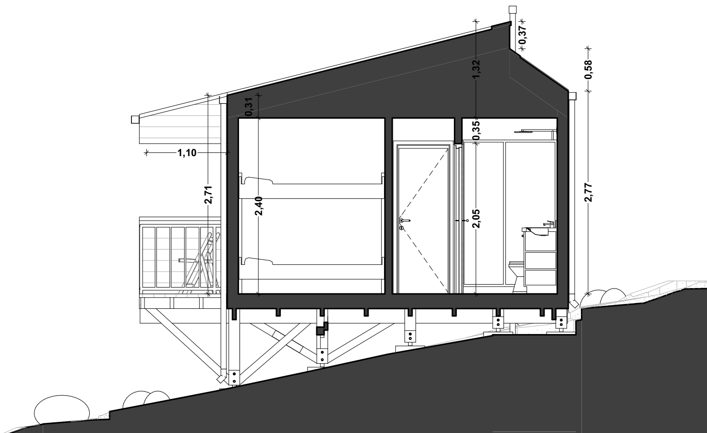
Corte C - C 1:50
