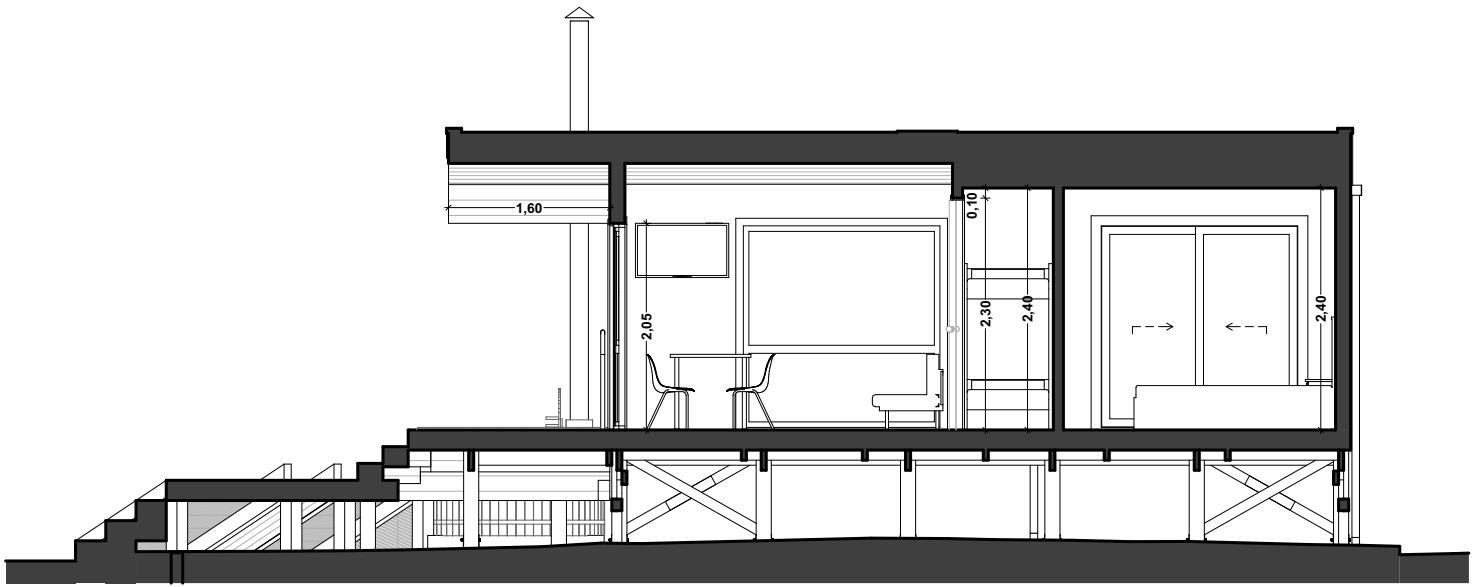
Corte F - F 1:75
