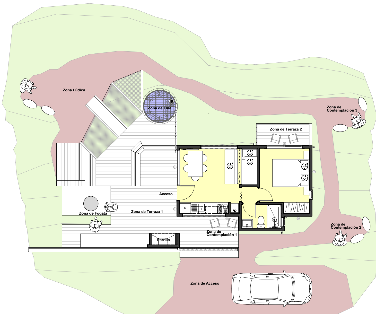
Planta de Arquitectura y Conjunto 1:100
