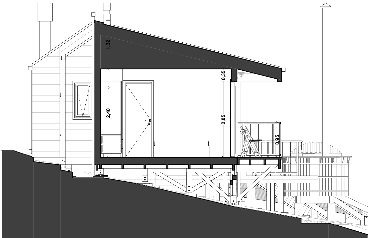
Corte E - E 1:50
