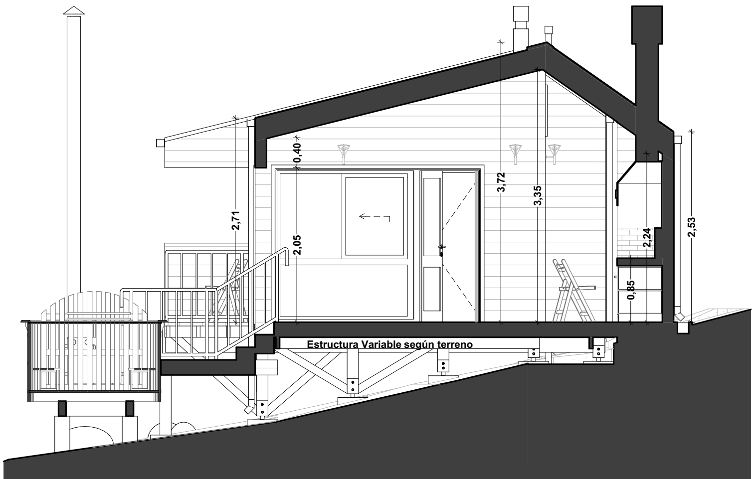
Corte A - A 1:50
