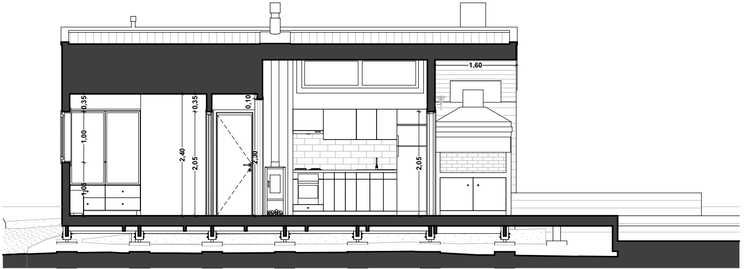
Corte G - G 1:75
